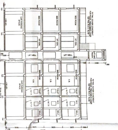
SECTION ON 'B-B' SCALE: 1:100
