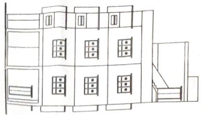
FRONT ELEVATION SCALE: 1:100
